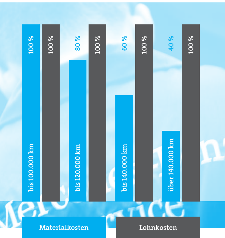
Materialkosten nach Betriebsleistung des beschädigten Bauteils
